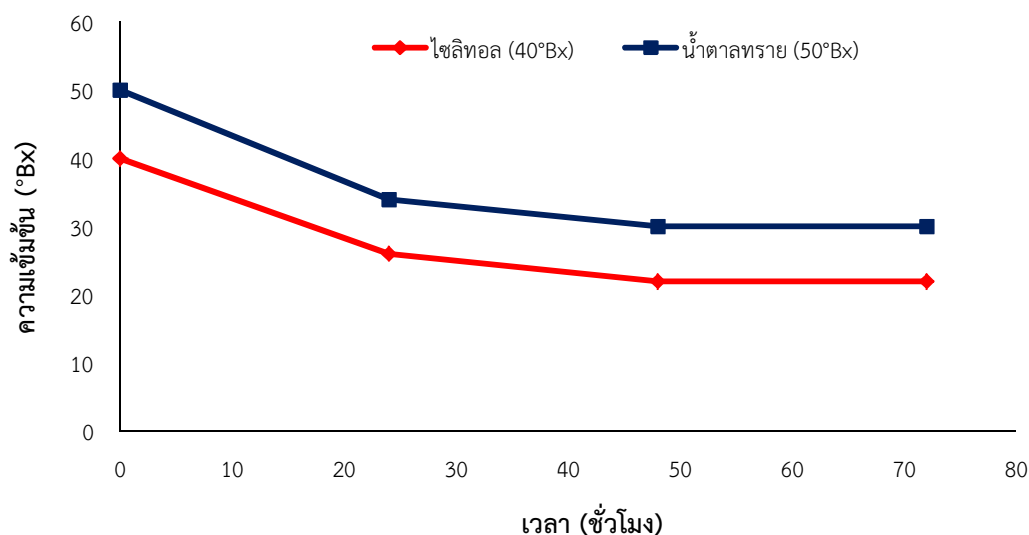
ภาพที่ 1.2 ความสัมพันธ์ระหว่างความชื้นน้ำเชื่อมกับเวลาในการแช่ขุ่นสววรรค์
